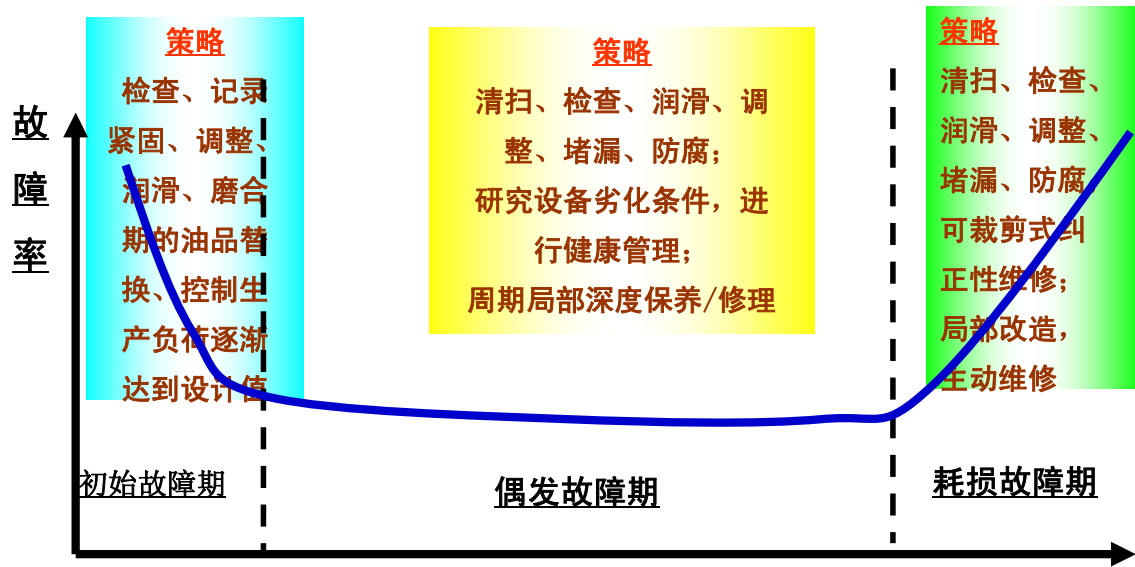
不同役龄区的维修策略安排
